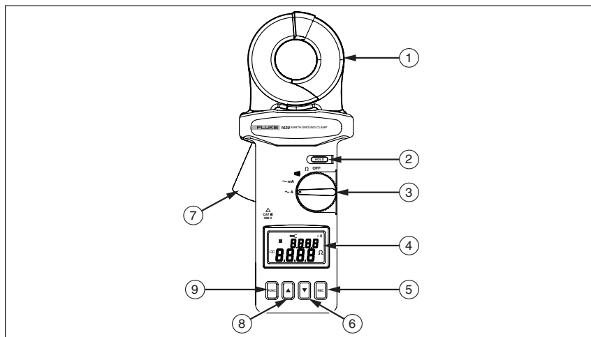
Obrázek 1. Funkce klešťového přístroje 1630
