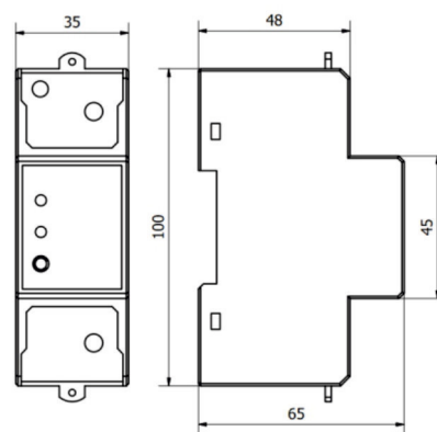
Dimensiones en mm - Dimensions in mm
