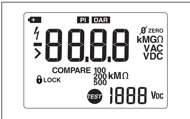
Obrázek 3. Symbyly displeje
