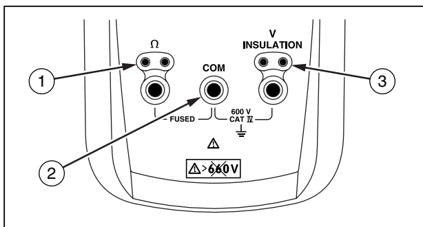
Obrázek 4. Vstupní zdířky
